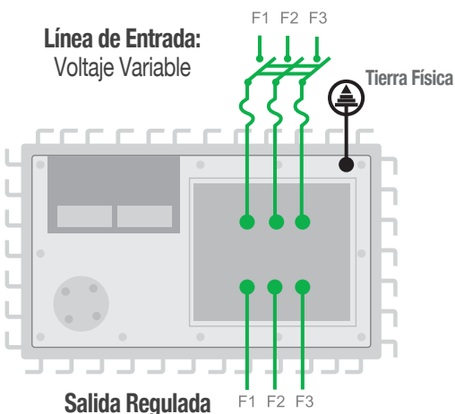
Sistema trifásico Delta
