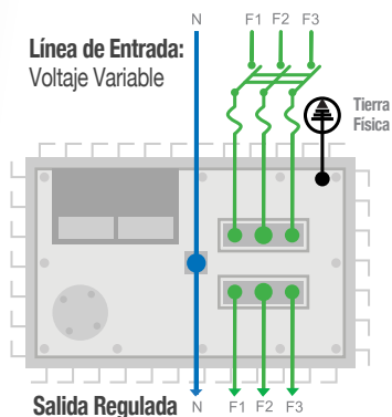
Sistema trifásico hasta 15kVA
