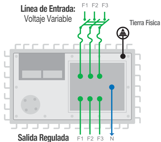
Sistema trifásico Delta / Estrella
