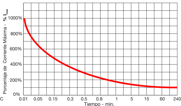
EN FUNCIÓN DE CONDICIONES DE SOBRECARGA ( I_{max} )
