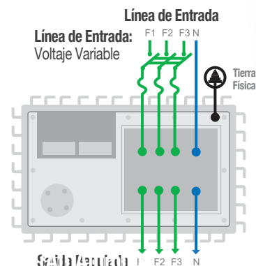
Sistema trifásico neutro independiente
