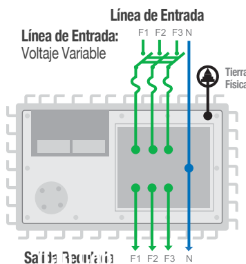
Sistema trifásico con neutro compartido
